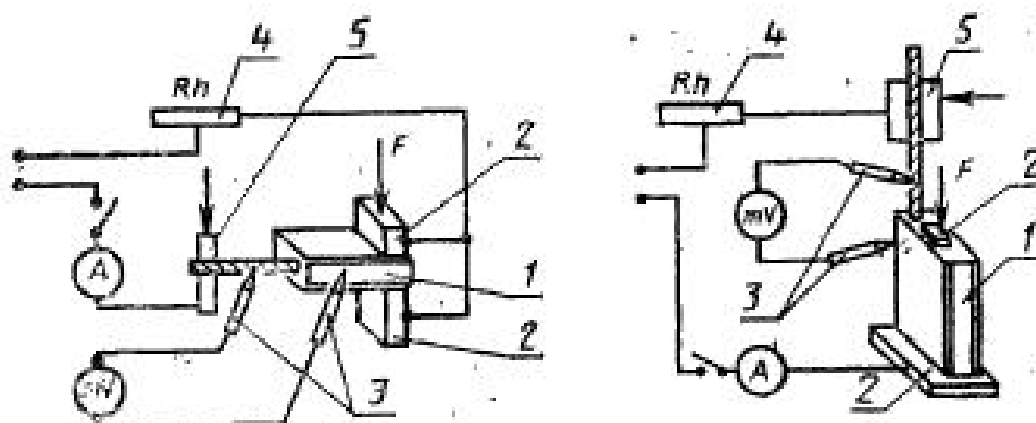
1 — щетка; 2 — зажимное устройство для щетки; 3 — угольные электроды; 4 — регулирующее устройство; 5 — зажимное устройство для провода
